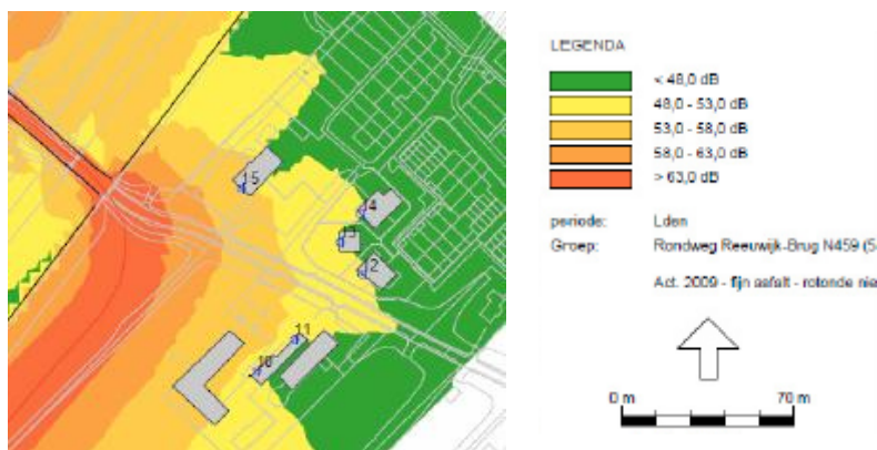
Figuur 6: Globale geluidscontour rondweg in 2020 zonder aanvullende maatregelen ter hoogte van de Nieuwdorperweg (excl. aftrek art. 110g Wgh) en inclusief beoordelingsposities omliggende woningen.
